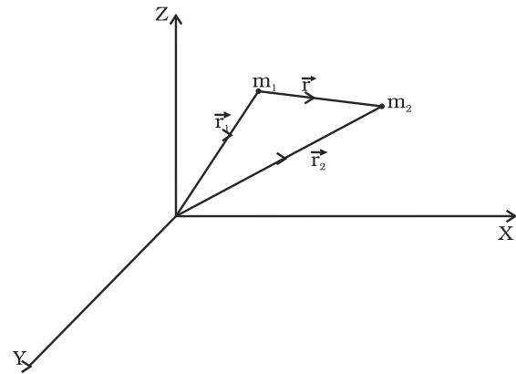
चित्र 8.3 m_2 के कारण m_1 पर गुरुत्वीय बल \mathbf{F} के अनुदिश है, यहाँ \mathbf{r}, (\mathbf{r}_2 - \mathbf{r}_1) है।
